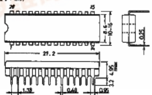
外形図 3029A-D2881C (unit: mm)
