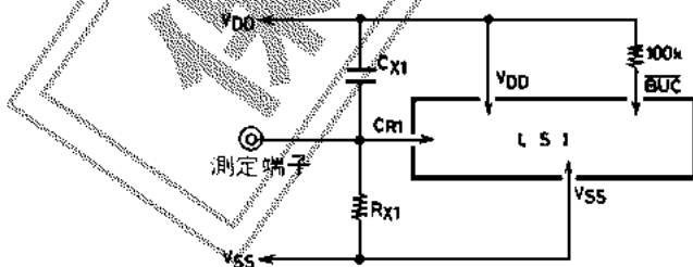
Fig 1 発振周期測定回路
