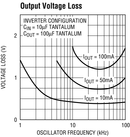
LT1054 • TPC07
