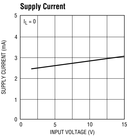
LT1054 • TPC02
