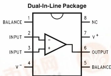
TL/H/5648-11
