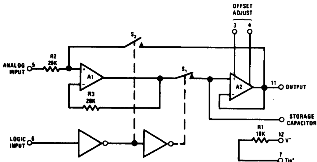
LH0023/LH0023C
