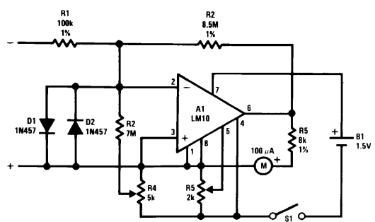
Meter Amplifier
