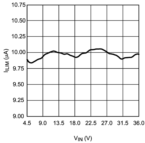
I_{LIM} vs V_{IN}
