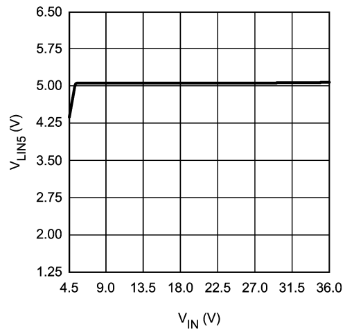
V_{LIN5} vs V_{IN}
