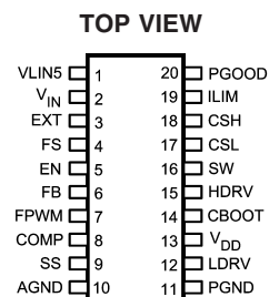
20-Lead TSSOP (MTC)
