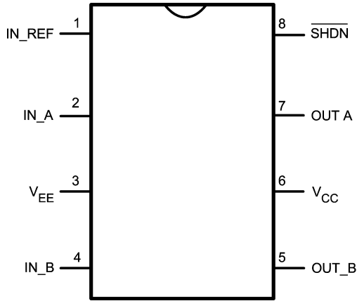
SOIC-8
