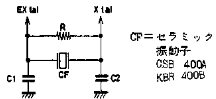
図2. 推奨発振回路
