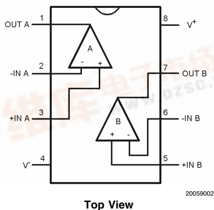
SOIC-8/MSOP-8 (LMH6682)
