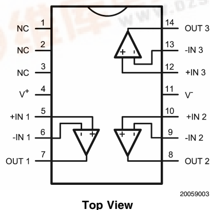
SOIC-14/TSSOP-14 (LMH6683)
