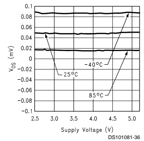
V_{OS} vs V^+
