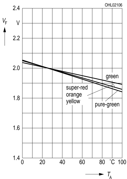
Durchlaßspannung V_F = f(T_A) Forward voltage I_F = 10 \text{ mA}
