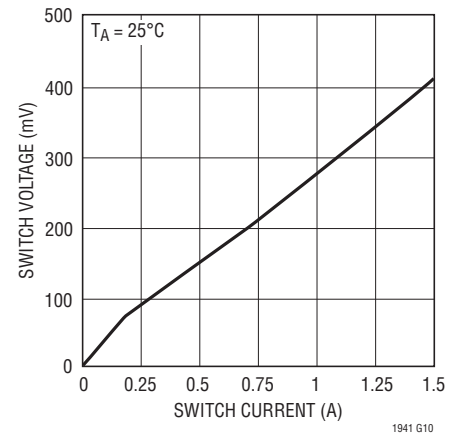
SW3 V_{CESAT}
