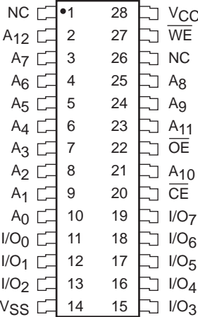
SOIC Package (J, K)
