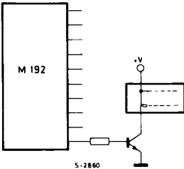
Fig. 4 - Incandescent readout
