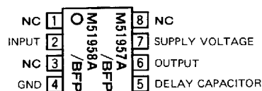
Outline 8P2S-A
