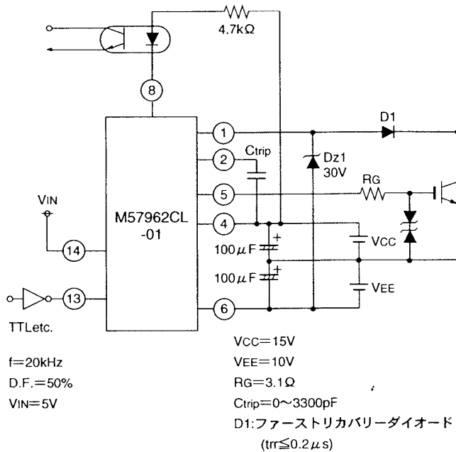
応用回路例
