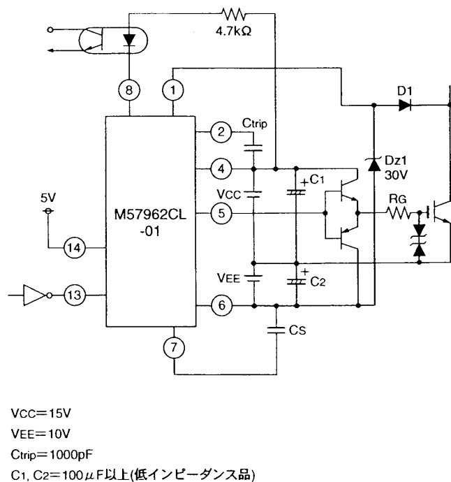
大容量素子の駆動回路例
