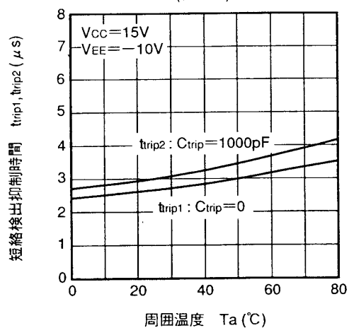
t_{trip1} , t_{trip2} — T_a 特性 (代表例)
