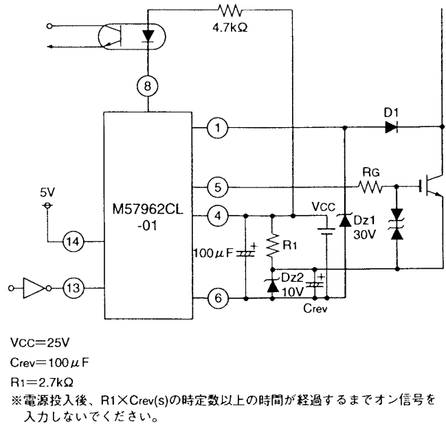
単電源使用回路例
