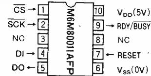
Outline 10P2N-A
