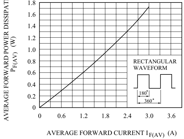
P_{F(AV)} - I_{F(AV)}
