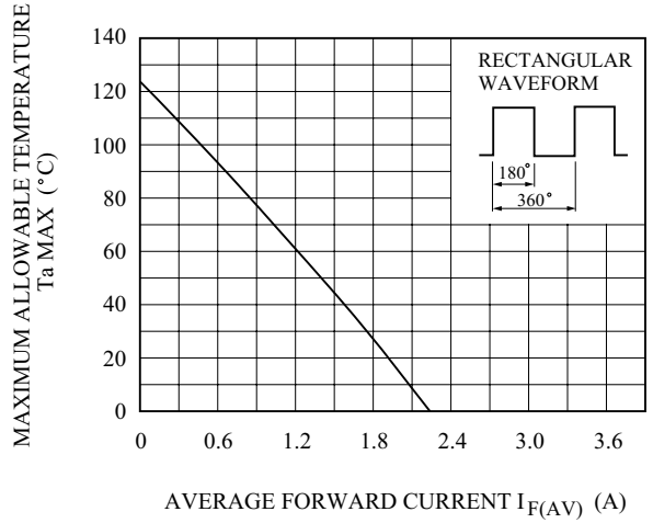
T_a - I_{F(AV)}
