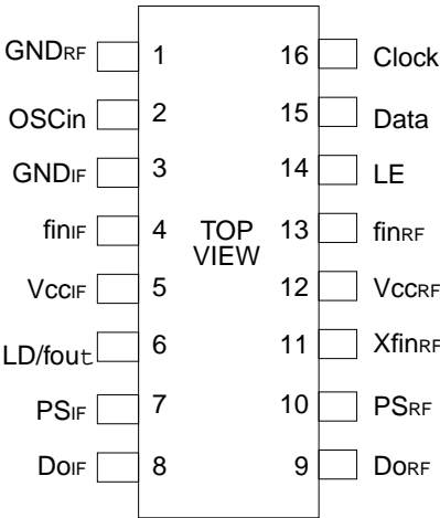
(FPT-16P-M05)
