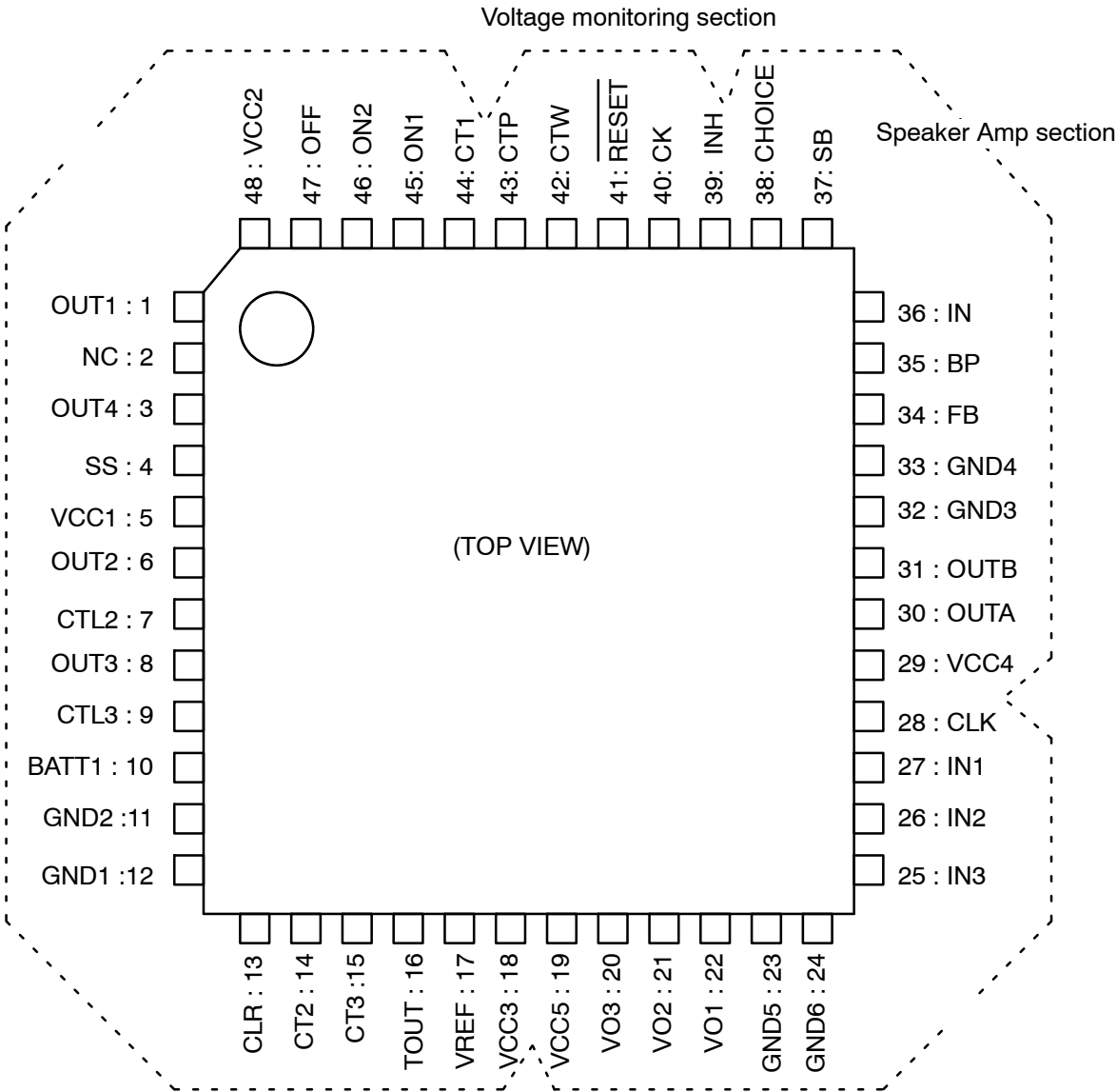
(FPT-48P-M05)
