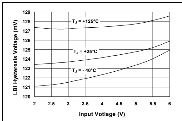
图 2-22: LBI 迟滞电压—输入电压曲线
