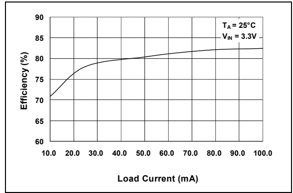
图 2-17: 效率—负载电流曲线
