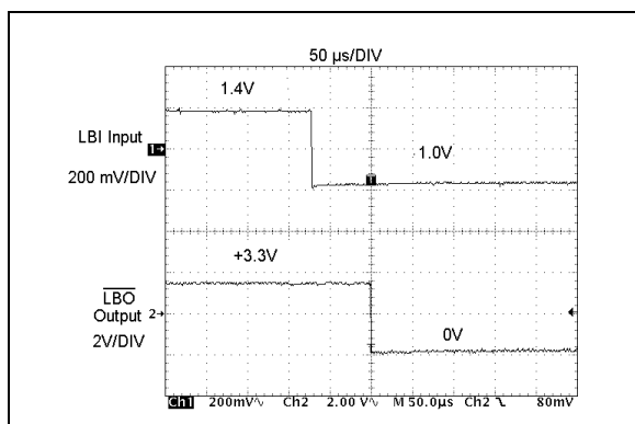
图 2-24: LBO 输出时序图
