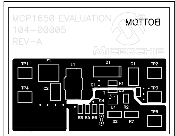
图 6-3: 底层走线
