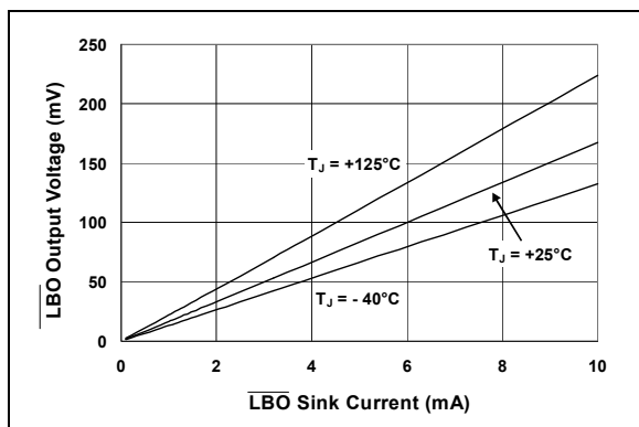
图 2-23: LBO 输出电压—LBO 灌电流曲线
