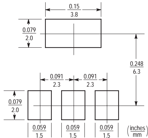
SOT-223
