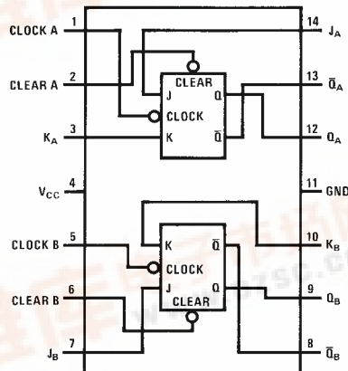
MM74C73
