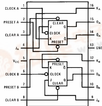
MM74C76
