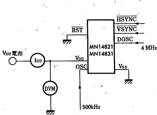
Fig. 3 電源電流 ( I_{DD} )測定回路
