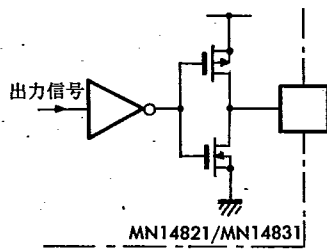
出力回路
