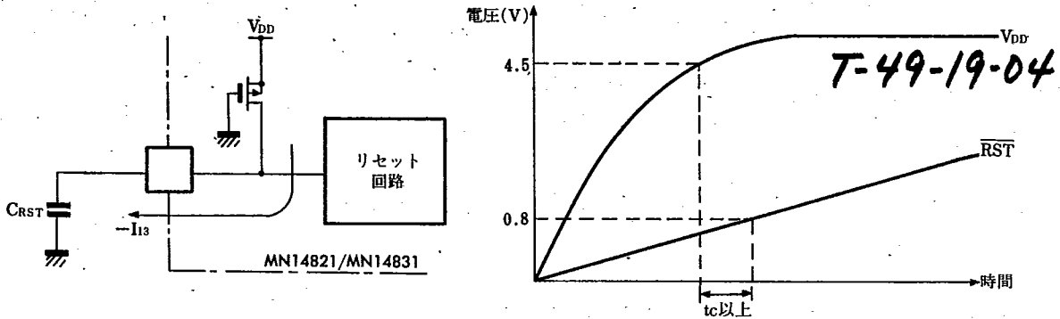
Fig. 7 イニシャルリセット回路および電圧波形
