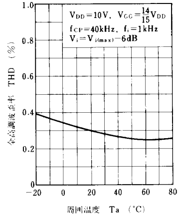
THD - T_a
