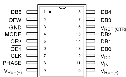
18 Pin SOIC (Jedec, 0.300")
