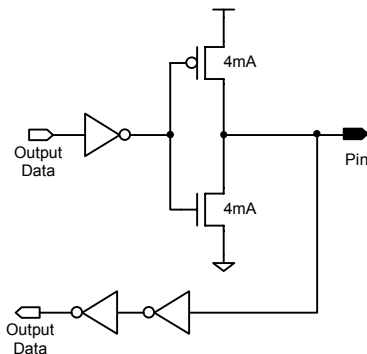
CMOS Pin (Output Mode) Pxxoe=1
