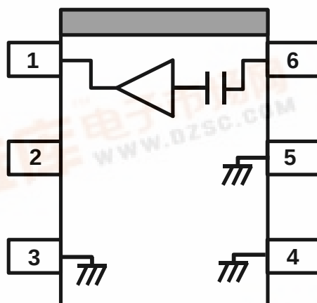
F1 TYPE (Top View)
