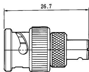
BNCP-MSSP CL311-0107-2
