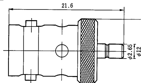
BNCJ-PO6J CL311-0167-4
