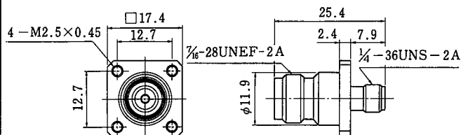
HRMJ-TNCJ-PA CL311-0202-3
