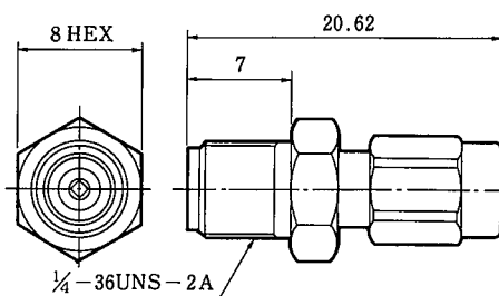
HRMJ-HRMMP-2 CL311-0221-8
