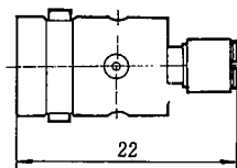
BNCJ-UMP CL311-0052-2
