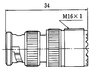
BNCP-MJ CL311-0008-0
