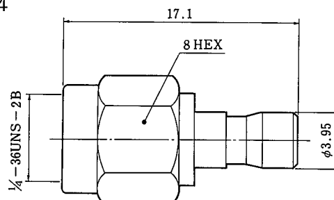
HRM.P-POD.J CL311-0177-8
