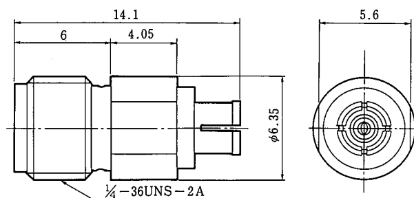
HRMJ-S.FLP CL311-0218-3
