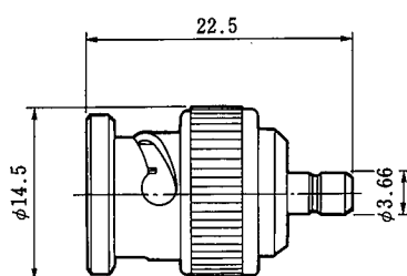
BNCP-UMJ CL311-0065-4
