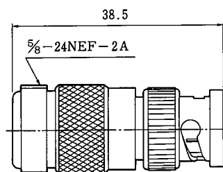
SJ-BNCP CL311-0060-0
