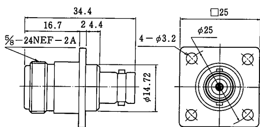
SJ-BNCJ-PA CL311-0108-5
