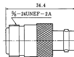
NJ-BNCJ CL311-0005-2
