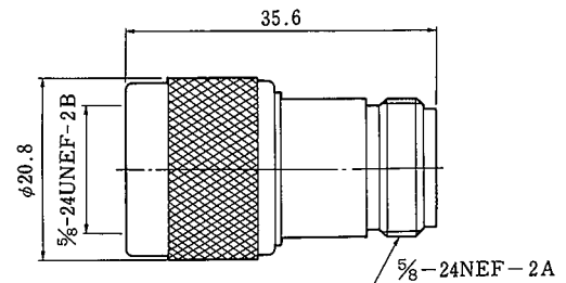
N.P-S.J CL311-0245-6
