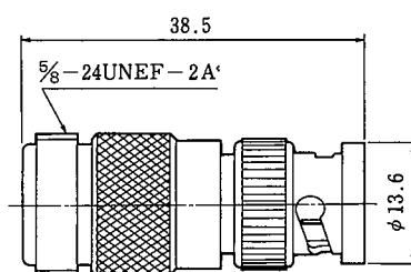
UG-349/U CL311-0004-0
