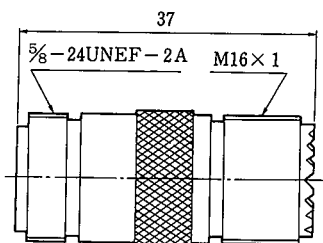
NJ-MJ CL311-0011-5
