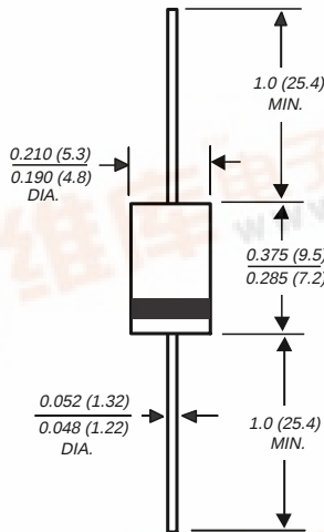
DO-201AD
