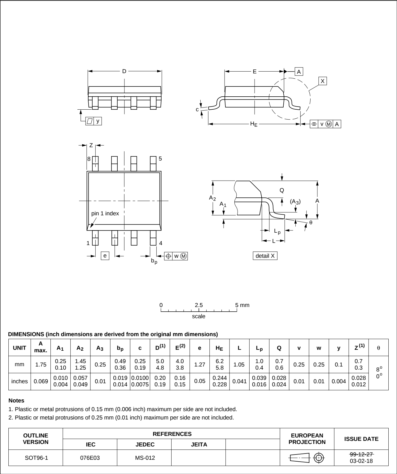
Fig 12. SOT96-1.
