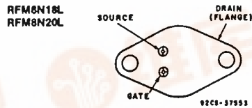
JEDEC TO-204AA
