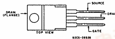
JEDEC TO-220AB
