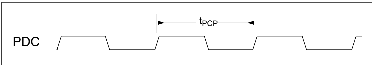
Figure 79 PDC Parameters
