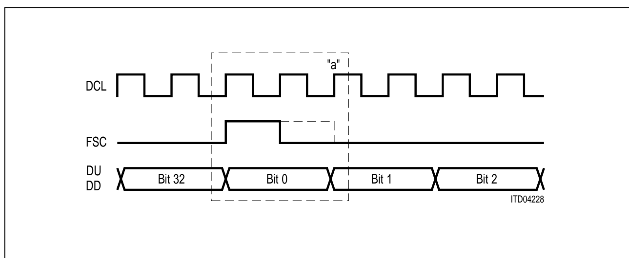
Figure 113 IOM ® -2 Interface Timing
