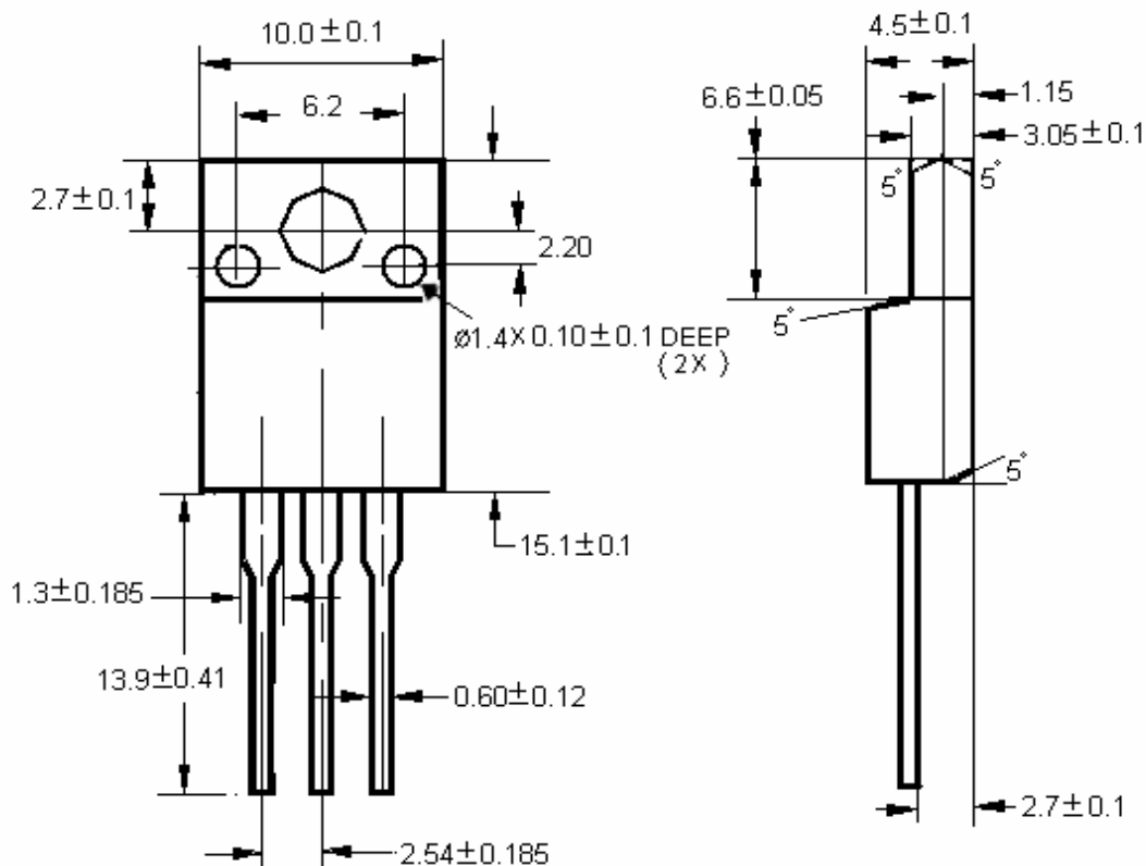
TO-220F Unit:mm
