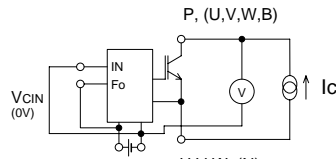
Fig. 1 V_{CE(sat)} Test
