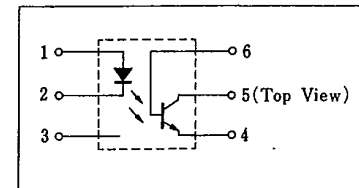
内部接続図 / Pin Connection
