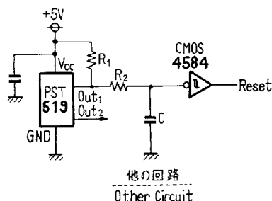
〔第4図〕 RESET パルス幅 が最小の動作例
