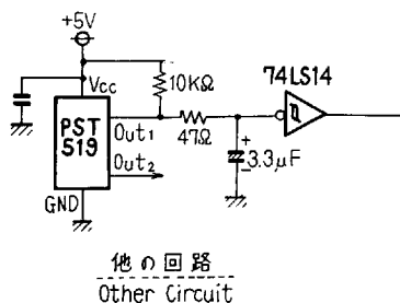
[Fig. 2] PST519 を用いたパワー・オンディレー回路/Power-ON delay circuit
