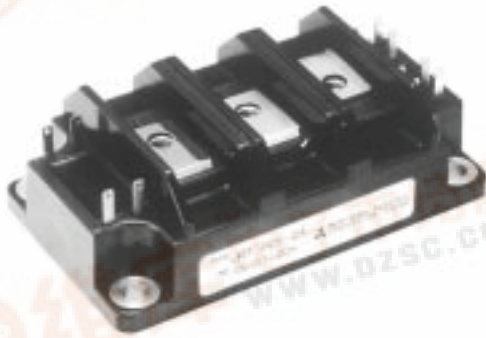
QM100DY-24BK
