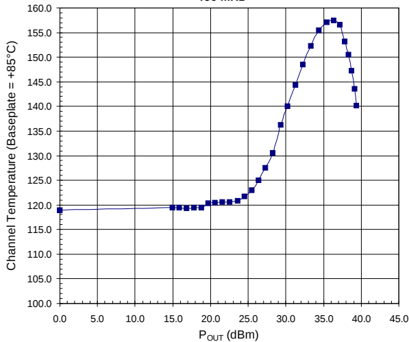
Thermal Data 460 MHz
