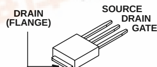
JEDEC TO-251AA
