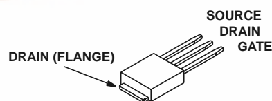
JEDEC TO-251AA
