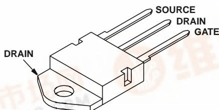
JEDEC TO-218AC
