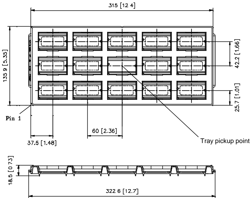
JEDEC TRAY
