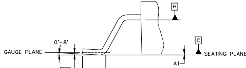
DETAIL "A" ROTATED 90° SCALE: B:1
