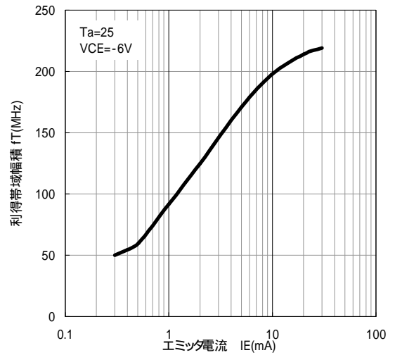
利得帯域幅積 - エミッタ電流
