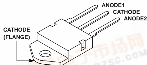
JEDEC TO-218AC
