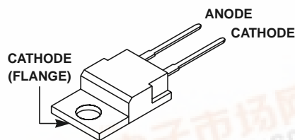
JEDEC TO-220AC
