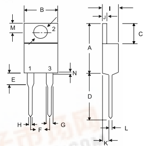
TO-220A
